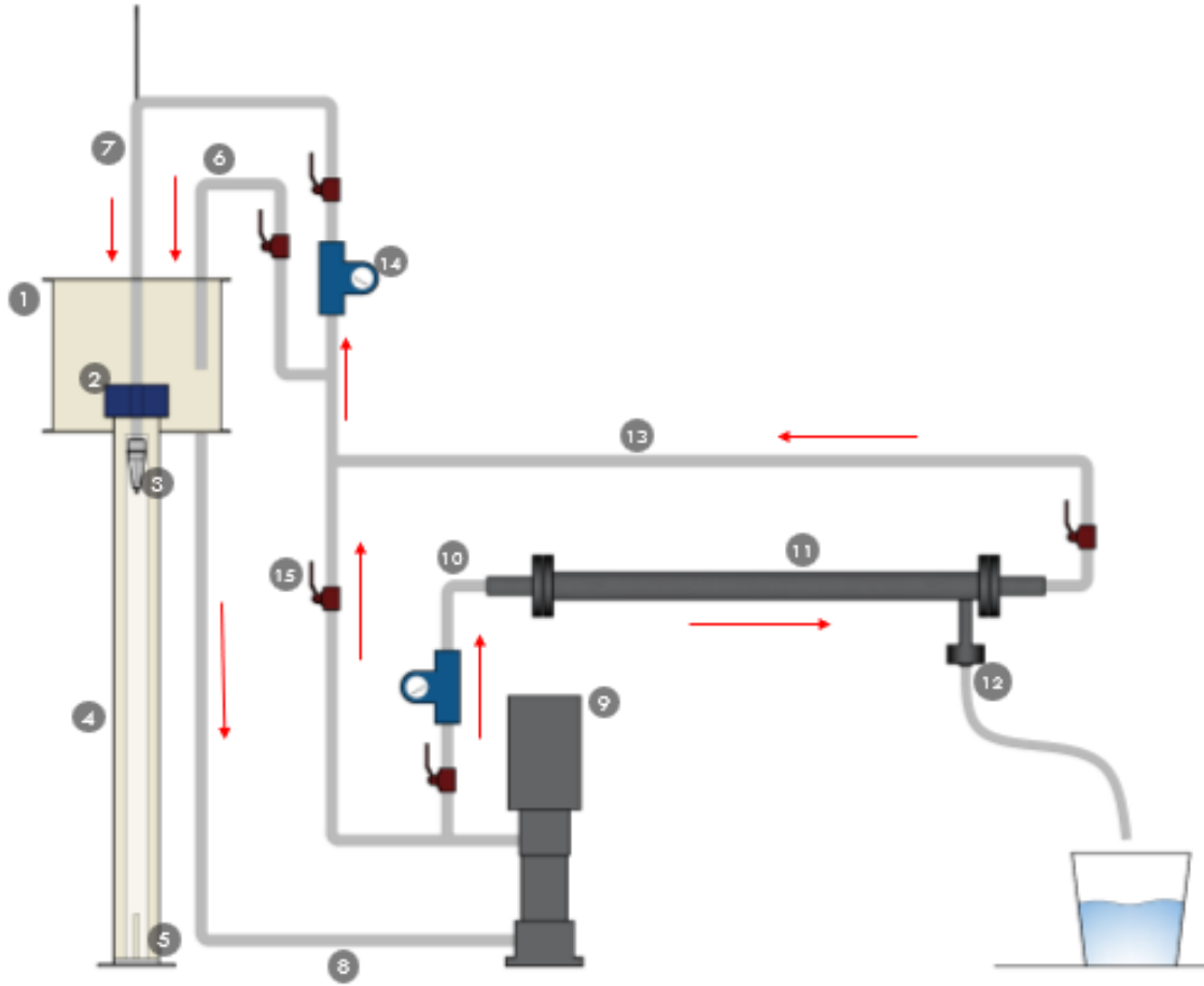
Şekil 3.3: Jet loop membran biyoreaktör (JLMBR) sisteminin akış şeması; 1: degazifikasyon tankı, 2: soğutucu 3: püskürtme başlığı (nozzle) 4: draft tüpü 5: çarpma levhası 6: by-pass hattı 7: reaktör besleme hattı 8: emme hattı 9: pompa 10: membran besleme hattı 11: seramik membran 12: membrandan çıkan süzöntü suyu 13: membrandan çıkan konsantre suyu 14: debimetre 15: vana
