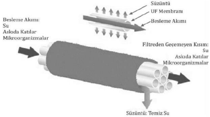
Şekil 2.13: Tübüler membran çalışma prensibi [9].
